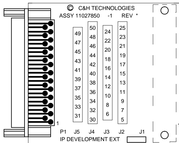
I/F EXTENDER/BREAKOUT LAYOUT
